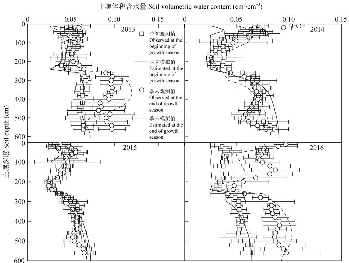
图 2 2013—2016 年六道沟流域 0~600 cm 剖面水分实测值与模拟值拟合程度对比
