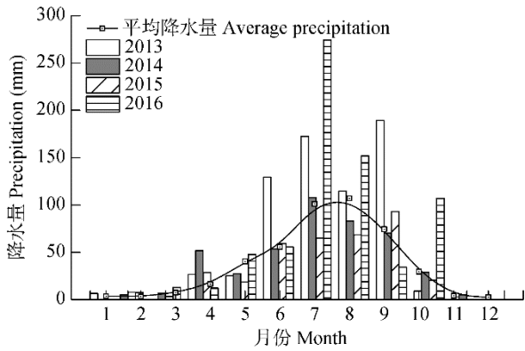
图 1 2013—2016 年六道沟流域月降水量分布和期间月平均降水量
