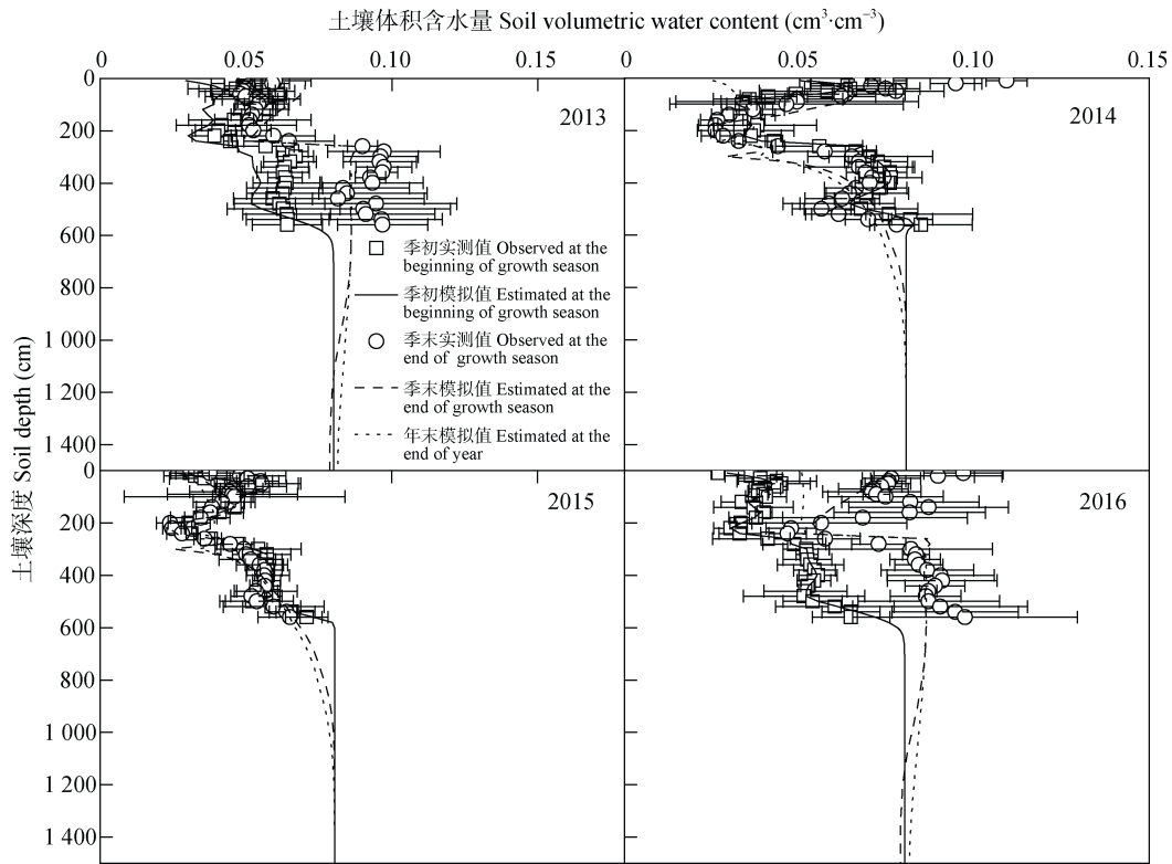
图 4 2013—2016 年生长季初、生长季末及年末的 1500 cm 深度水分分布的模拟结果
