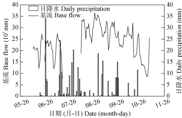
图 5 2015 年临近试验区的沟道基流与日降水变化
